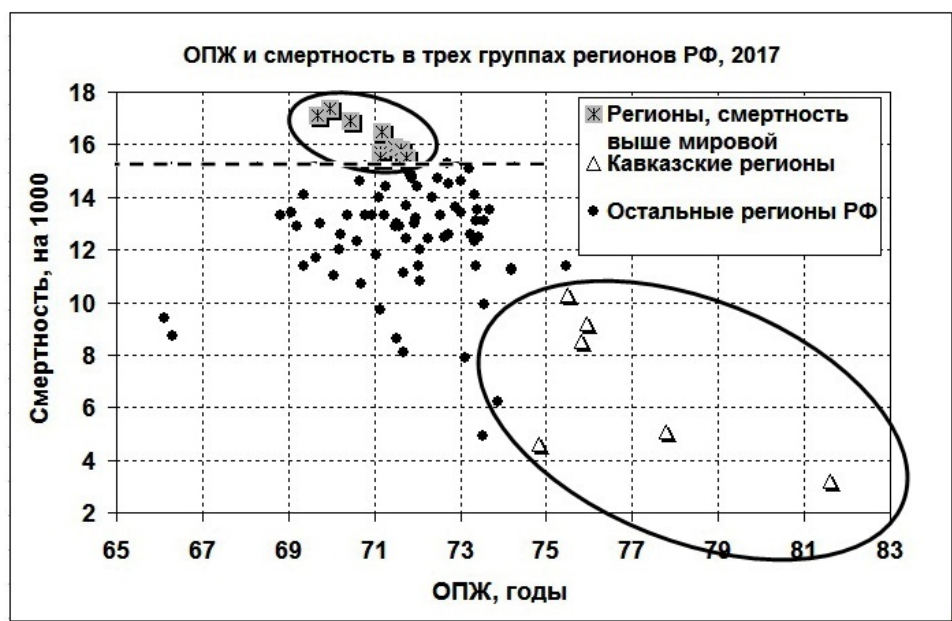
Рис. 2. Связь ожидаемой продолжительности жизни (ОПЖ) и общей смертности населения регионов России в трех группах регионов в 2017 г. Объяснения в тексте. Штриховая линия указывает положение максимальной смертности стран мира в 2017 г.
