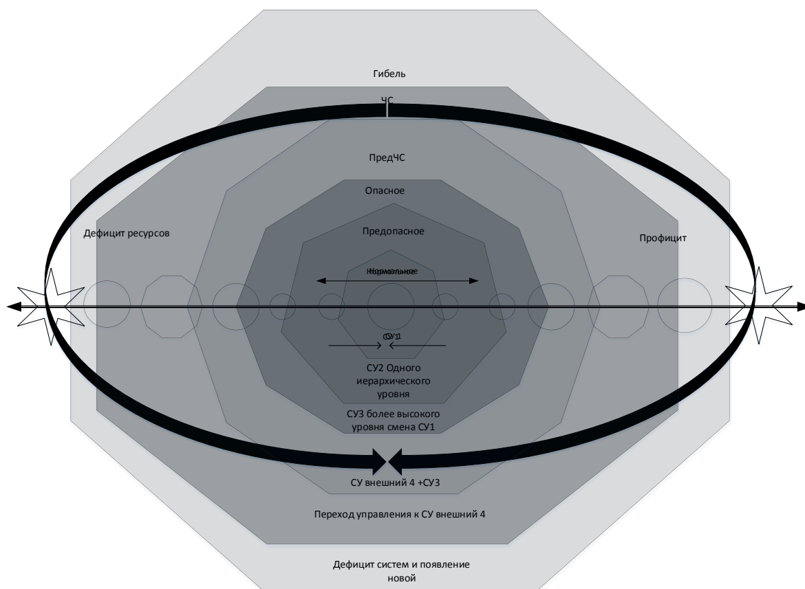
Рис. 1. Вариант отображающей оси функциональной аттракции в пределах фуркационных значений обобщенного параметра
