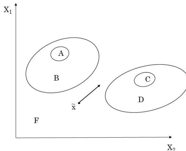
Рис. 2. Возможная картинка в фазовом пространстве. А и С — аттракторы, В и D — их области притяжения, F — точка, соответствующая начальному состоянию системы \tilde{x}
