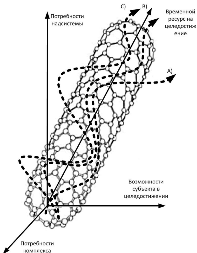
Рис. 2. Вариант фазового пространства функциональной аттракции динамической системы в пределах фуркационных значений обобщенного параметра
